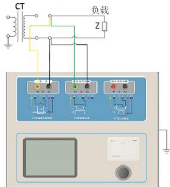
图 2-2 CT 二次负荷试验接线图
